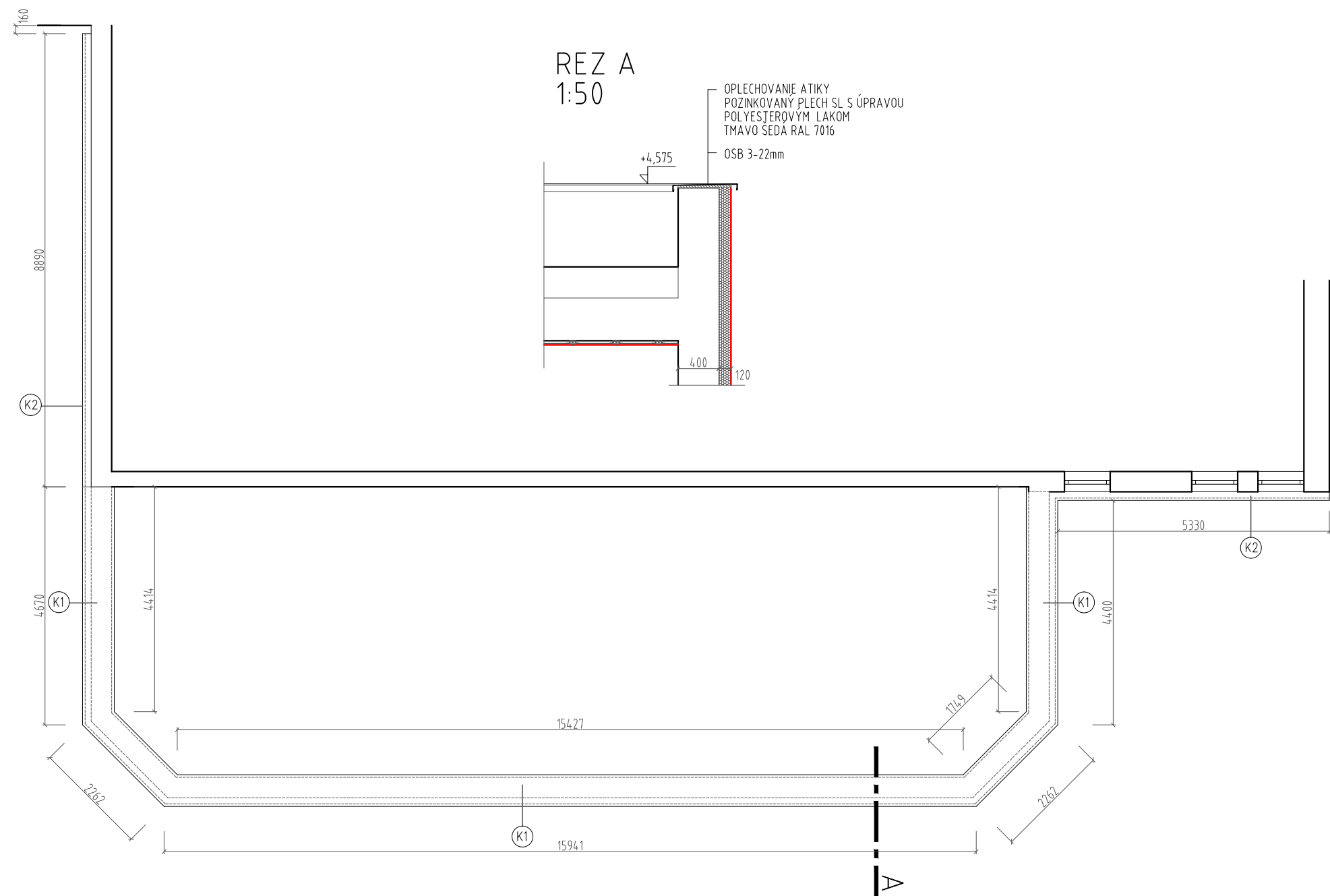
Oplechovanie atiky
